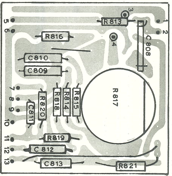
POTENTIOMETERPLAAT PLAQUE DE POTENTIOMÈTRE
